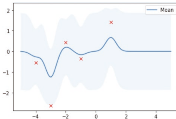
Figure 2-16. GP posterior using optimized kernel parameters
